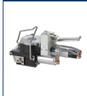
Flejadora ITI - 14
